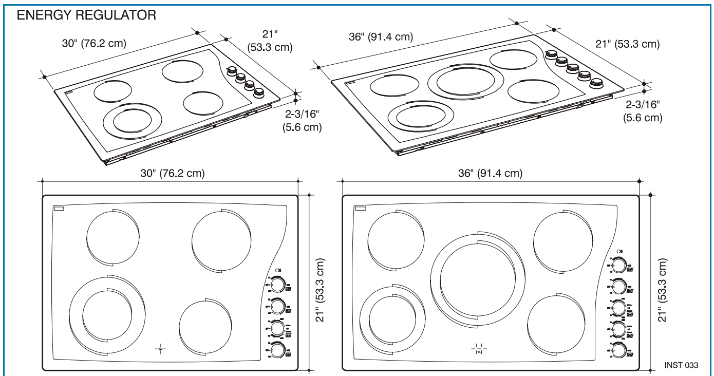
Figure 2. Régulateur d'énergie (Energy Regulator)
